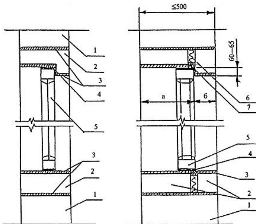
Вариант с многослойной перегородкой
